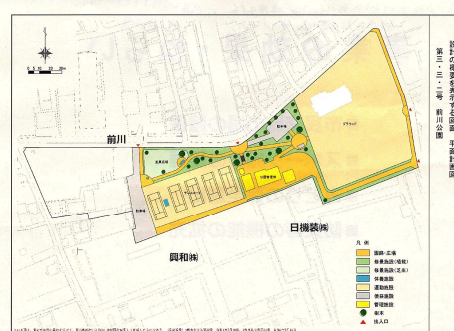
平面図計画図
